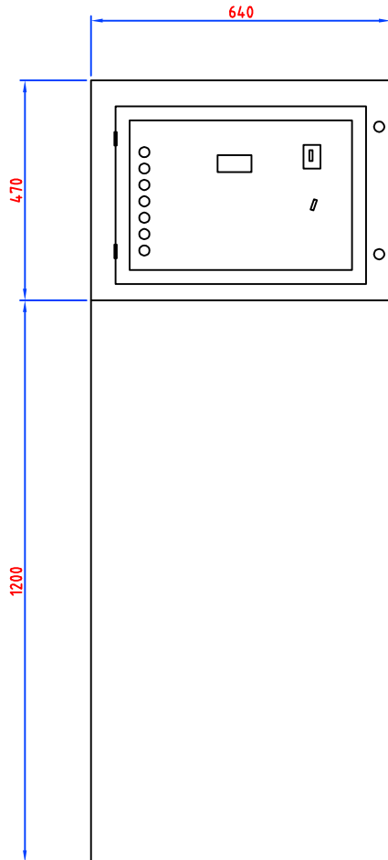
Gearceerde gedeelte is de beschikbare ruimte tbv mantelbuizen
