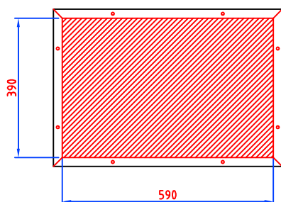
Gearceerde gedeelte is de beschikbare ruimte tbv mantelbuizen
